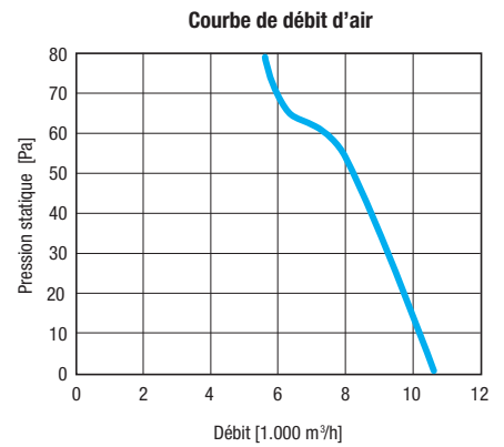
Graphique pour moteur ED24 3Ph 50 Hz multivitesse. Extracteur testé avec volet et grille de protection.
