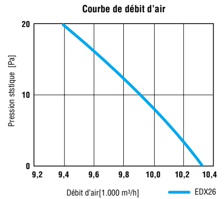
Courbe du modèle EDX26 à moteur 50 Hz triphasé.
